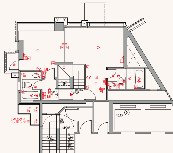
UPPER PART OF DUPLEX UNIT 複式住宅單位上層 21/F, 42/F 二十一樓及四十二樓
