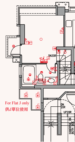
UPPER PART OF DUPLEX UNIT 複式住宅單位上層 7/F 七樓
