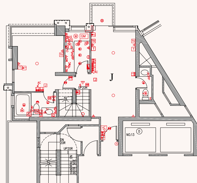
LOWER PART OF DUPLEX UNIT 複式住宅單位下層 23/F 二十三樓
