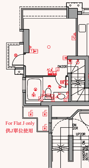
UPPER PART OF DUPLEX UNIT 複式住宅單位上層 25/F 二十五樓
