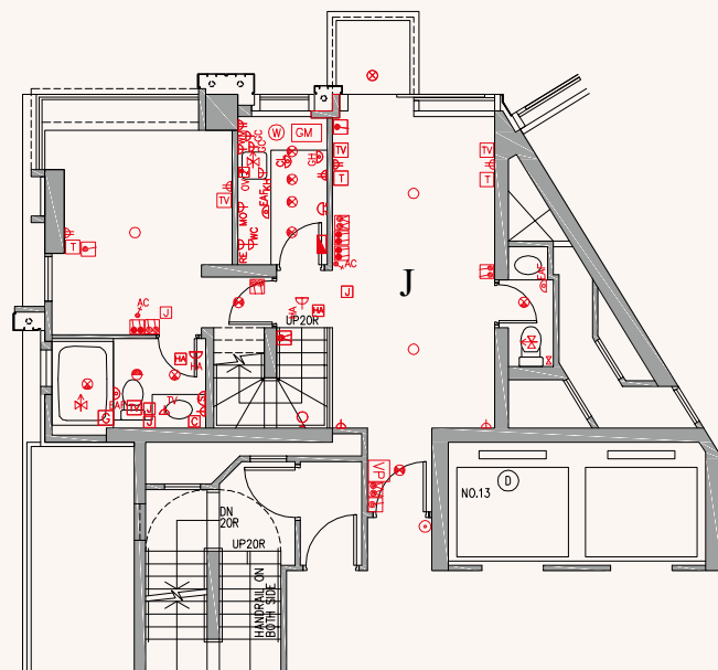
LOWER PART OF DUPLEX UNIT 複式住宅單位下層 6/F 六樓
