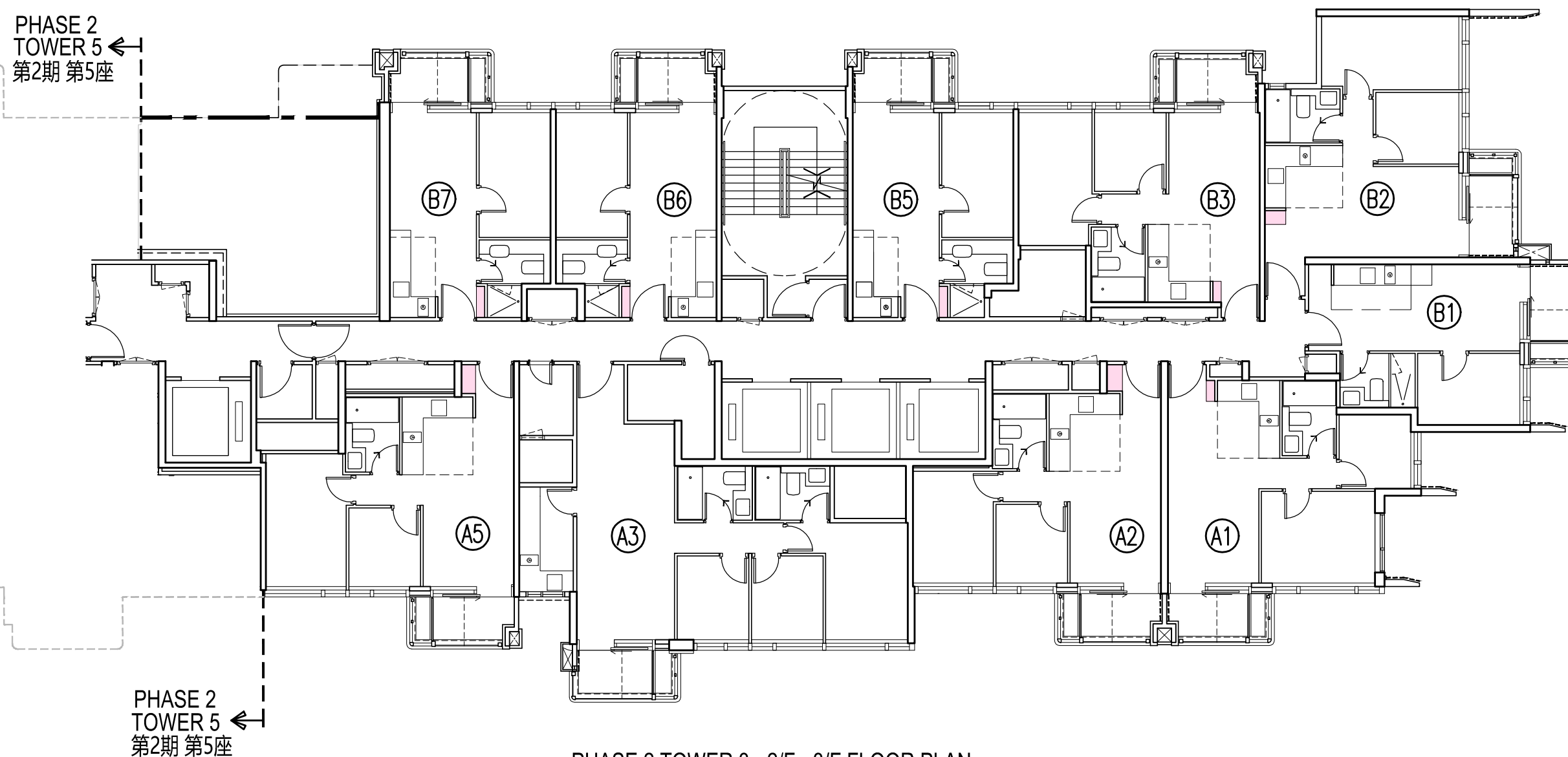
PHASE 2 TOWER 3 - 2/F - 3/F FLOOR PLAN 第2期第3座 - 2樓-3樓 樓面平面圖
