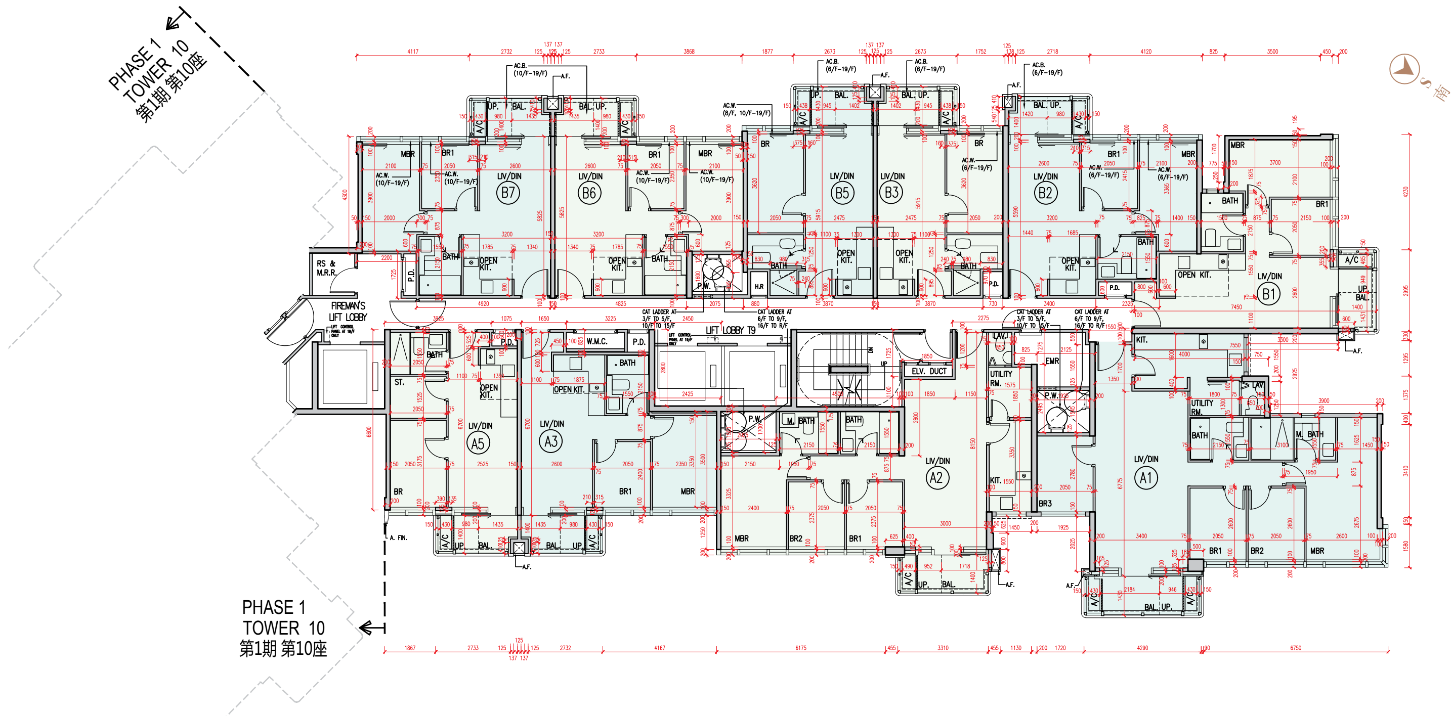
Key Plan 指示圖
