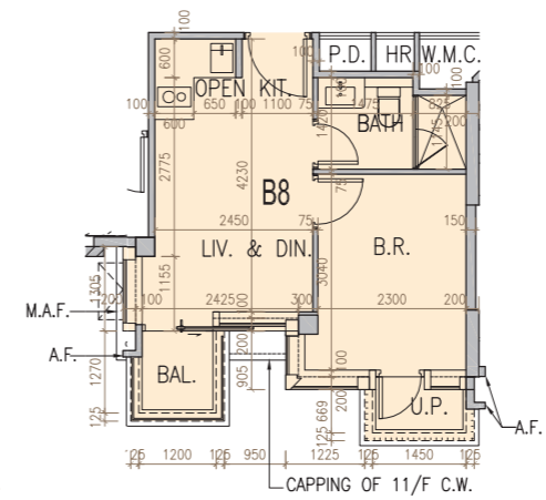
12/F part plan 12樓部份樓面平面圖
