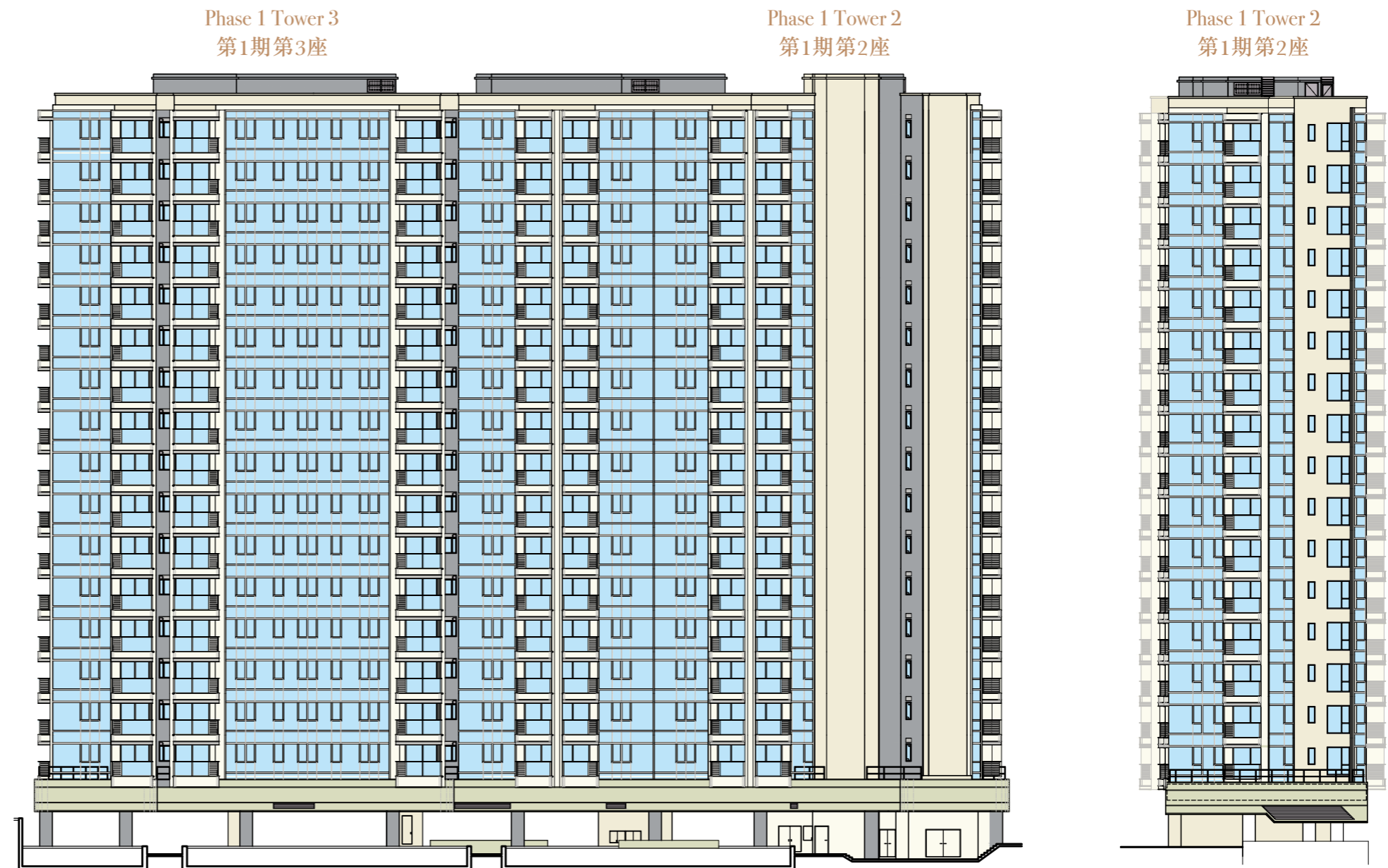
Elevation C 立面圖 C
